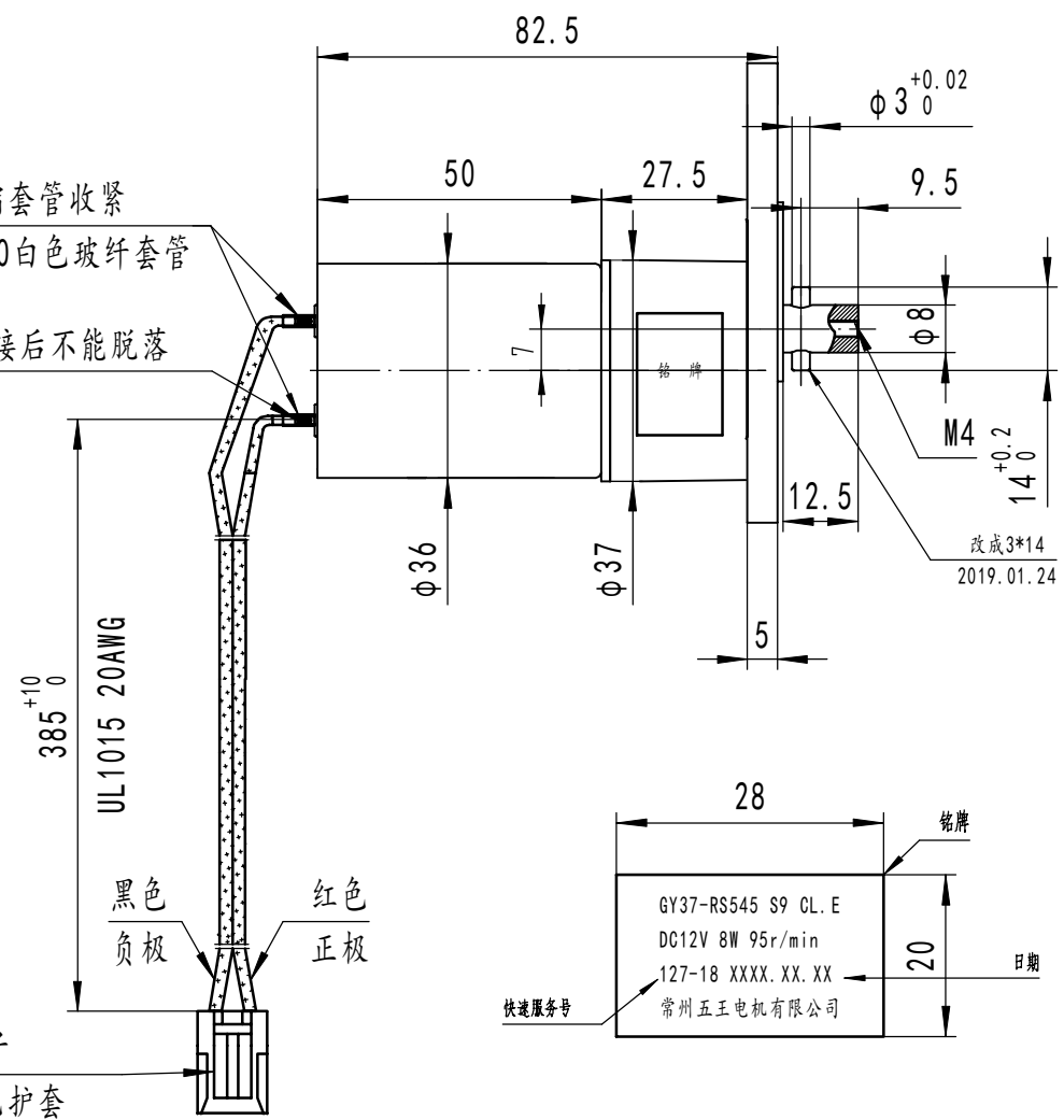
电机外形图
